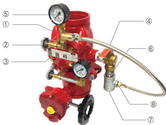
C-TYPE 드레인밸브
