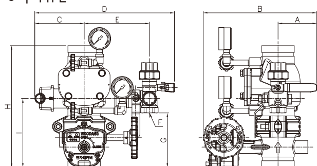
C-TYPE 드레인 밸브
