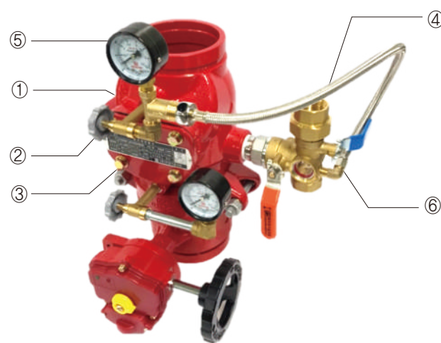
U-TYPE 드레인밸브
