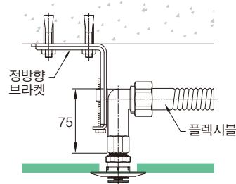
정방향 브라켓 : 플렉시블과 반대 방향
